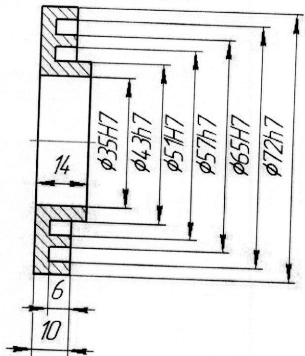
Деталь №2
