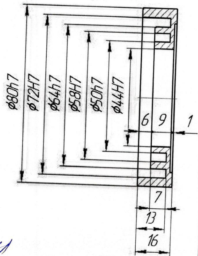
Деталь №1
