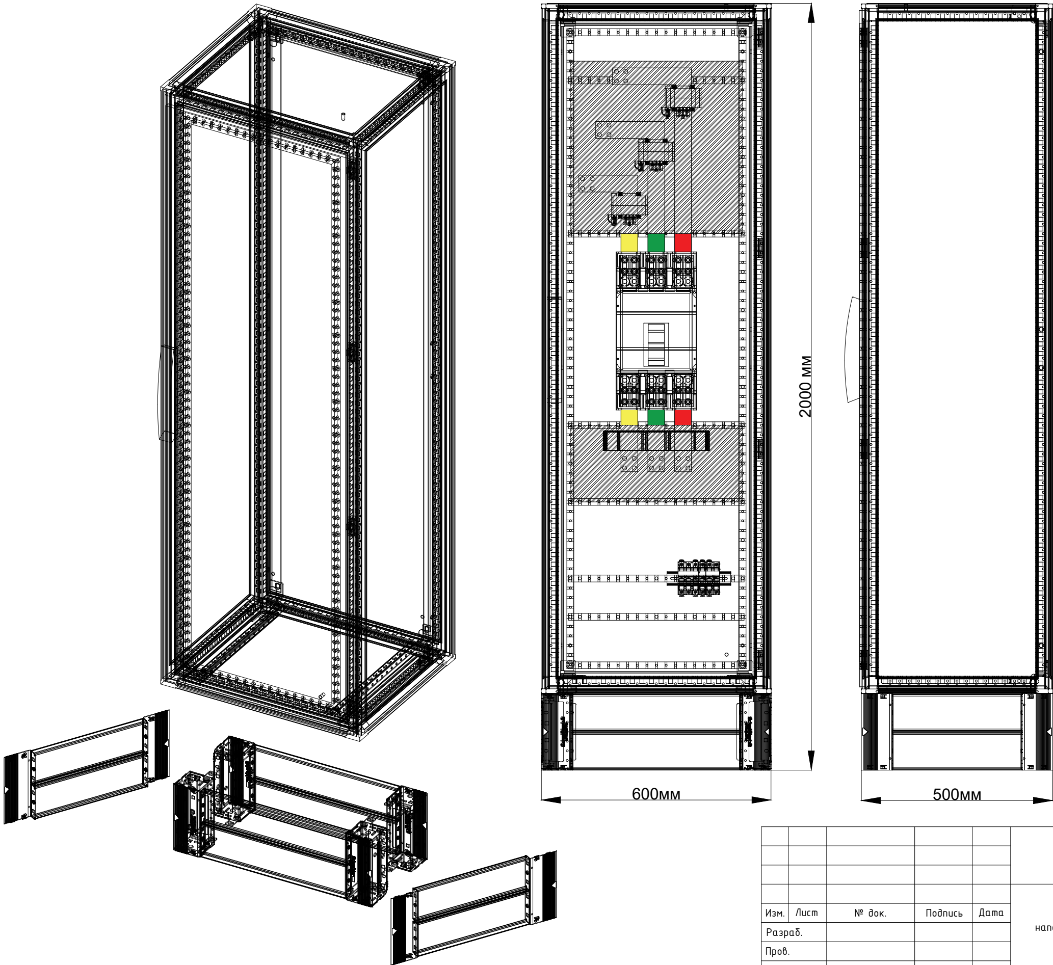
Расположение оборудования на монтажной панели
