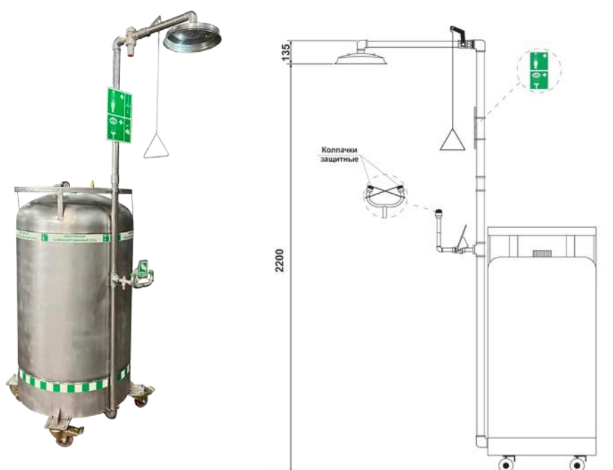
Рис.1 Аварийный комбинированный передвижной автономный душ
