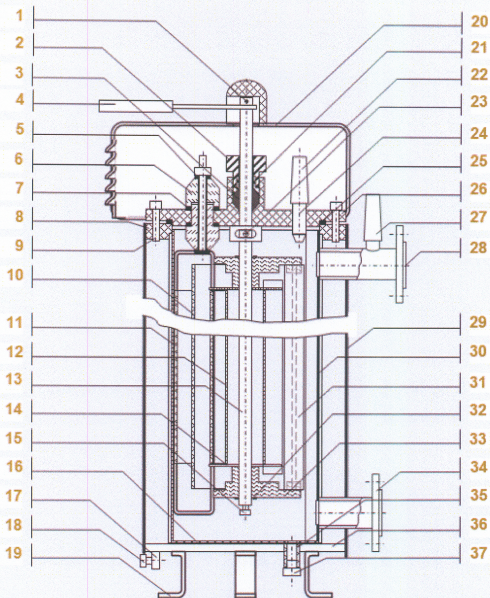
Рис. 3 Устройство электроводонагревателя
