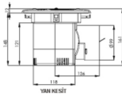
YAN KESİT
