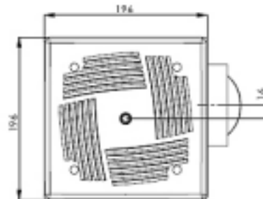
ÜST KESİT
