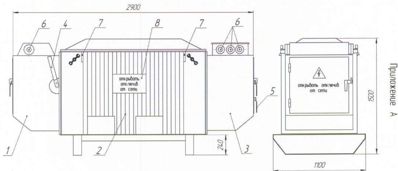
Рис. 1 Общий вид и габаритные размеры подстанции КТПШГ.
