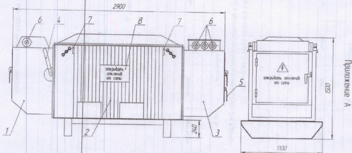
Рис. 1 Общий вид и габаритные размеры подстанции КТПШГ.
