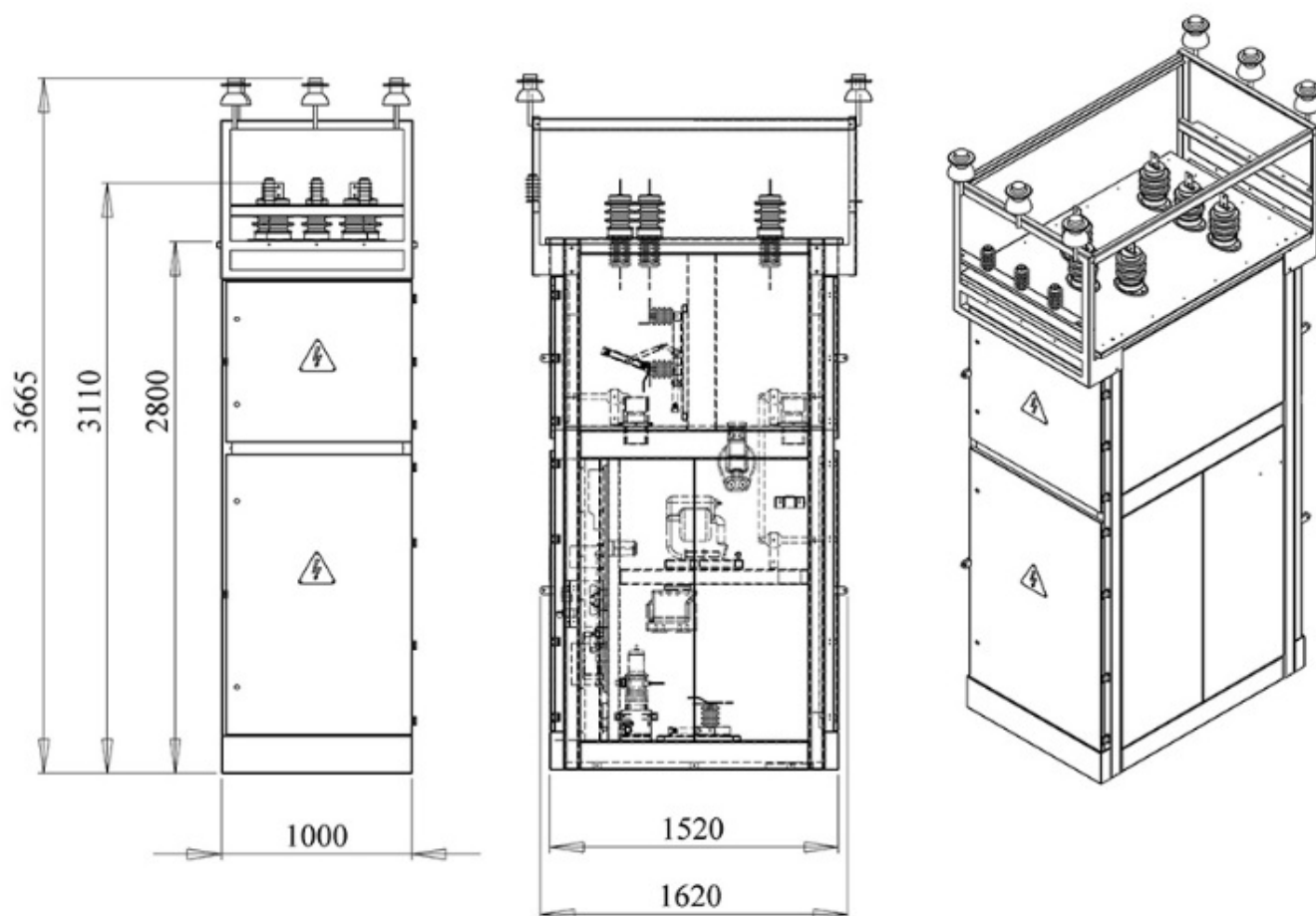
ЯКНО-К/К (кабель-кабель)
