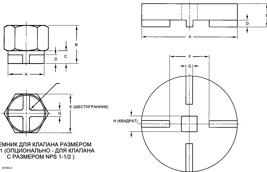
Рис. 7. Данные для изготовления и использования съемника фиксатора (поз. 33) (см. также табл. 6 и 7)
