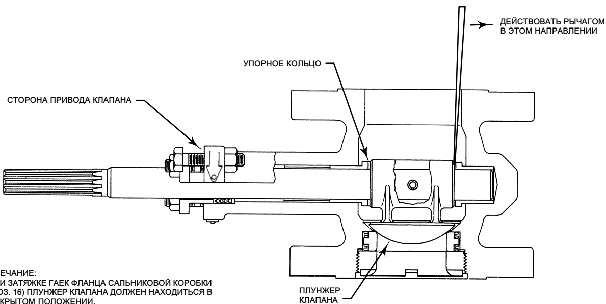
Рис. 6. Использование монтировки
