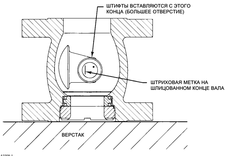
Рис. 10. Детализировка плунжера клапана для установки штифта
