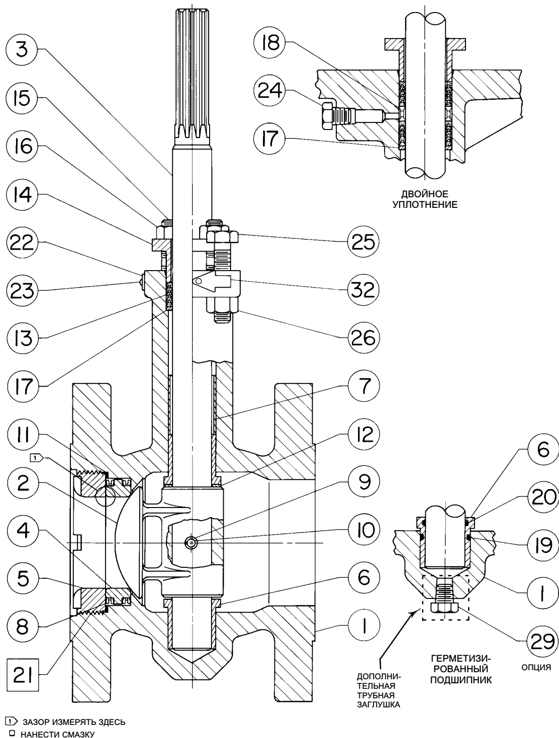
Рис. 13. Поворотный регулировочный клапан V500, NPS 2, 3, 4, 6 и 8
